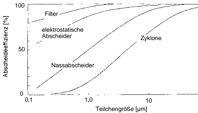
Vergleich der Abscheideeffizienz verschiedener Systeme
