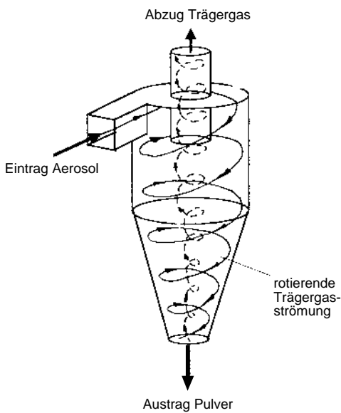
Pulverabscheidung im Zyklon
