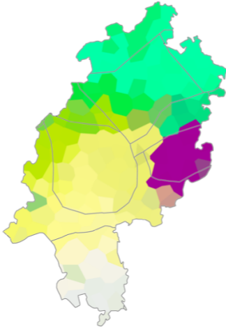
Gesamtkarte: Syntaxdaten
