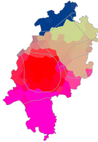
Gesamtkarte: N-Gramm-Daten
