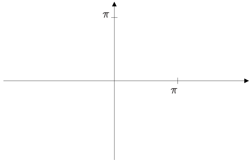
Reziprokes Gitter
