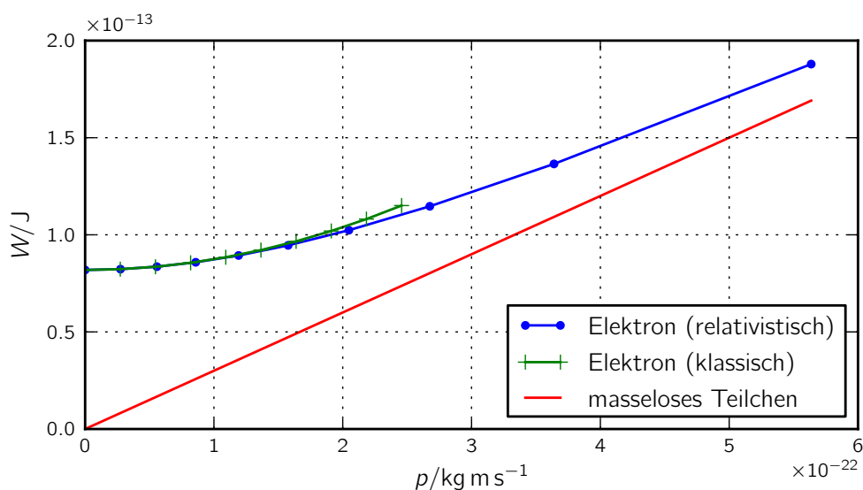
Abbildung 1: Energie-Impuls-Diagramm.
