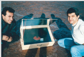
Test des selbstgebauten Solarkochers 1995
